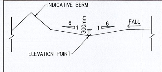
TYPICAL DRAIN CROSS SECTION (D) SCALE 1:20
